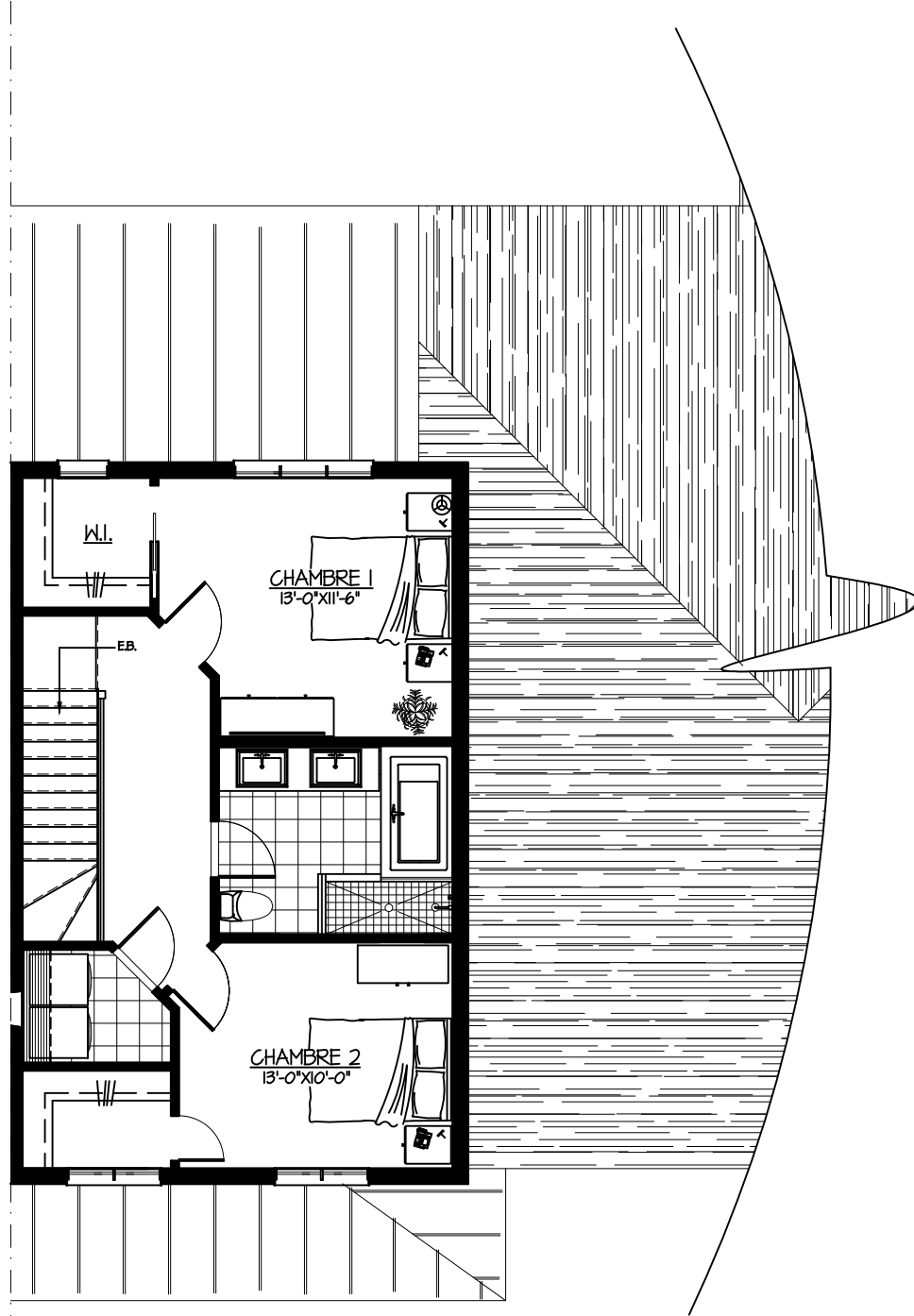
PLAN DE L'ETAGE SUPERFICIE COTTAGE DROITE : 630 PI CA.
