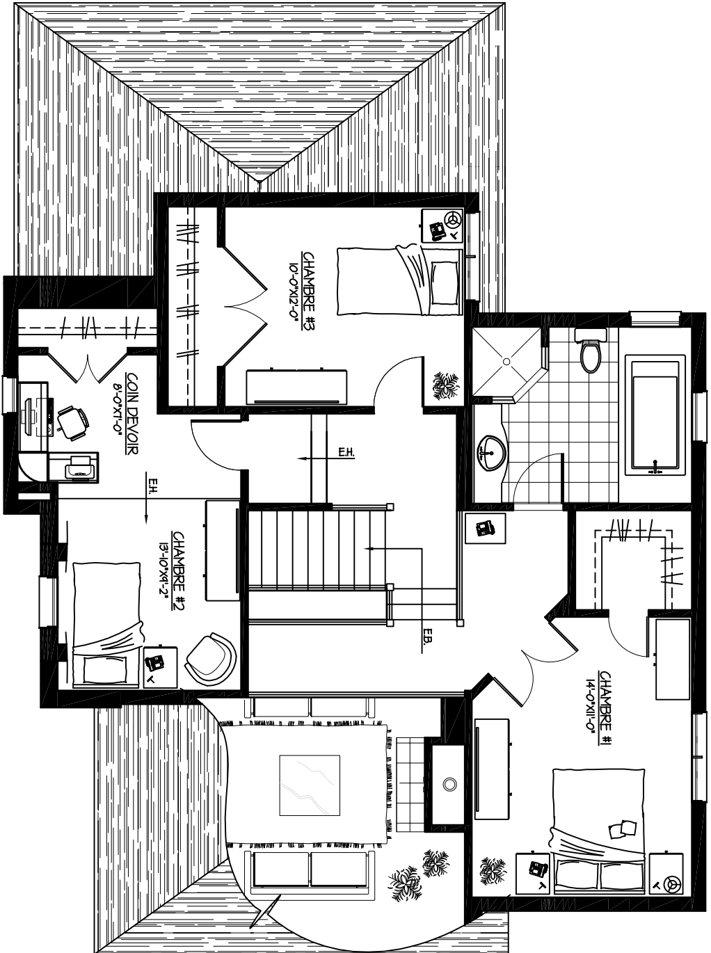
PLAN DE LETAGE SUPERFICIE : 874 P.I.C.A.
